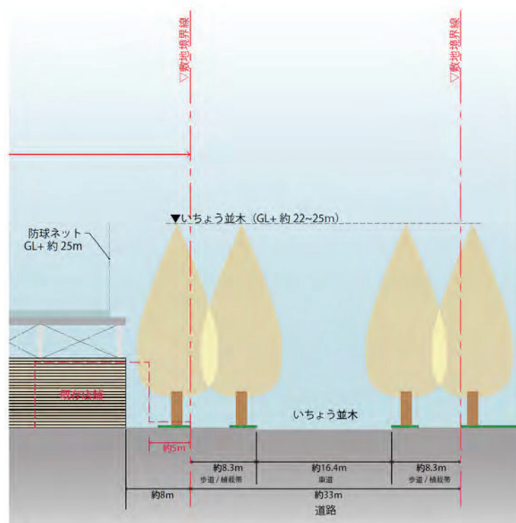
図2.7-1(1) いちよう並木西側（野球場）の断面イメージ
