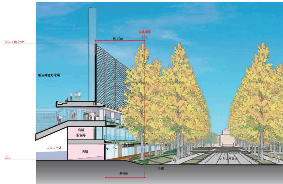
図2. 7-2 眺望の状況（青山二丁目交差点付近）
