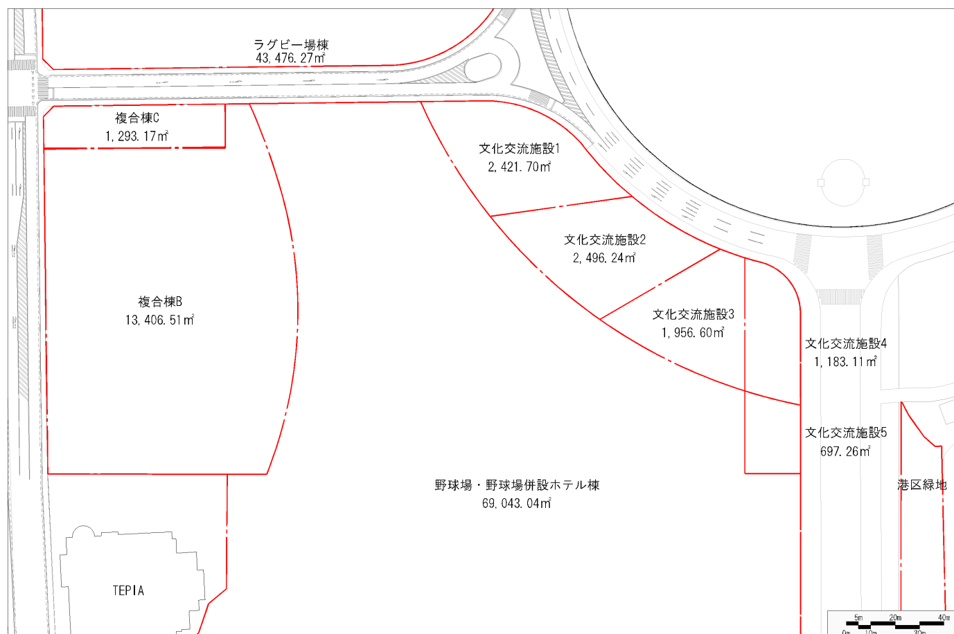
神宮外苑地区第一種市街地再開発事業 配置設計図 施設建築敷地図
