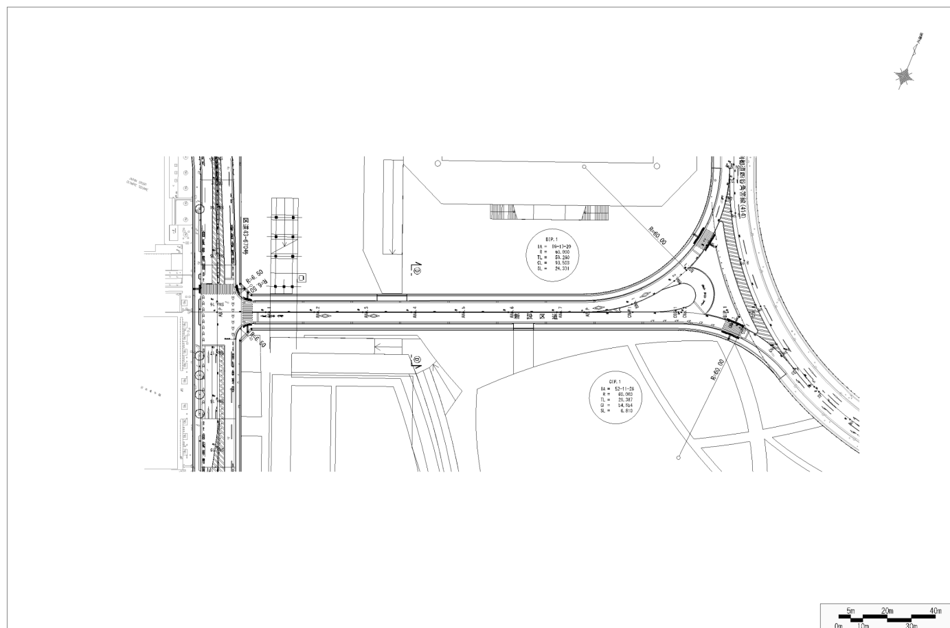
神宮外苑地区第一種市街地再開発事業 配置設計図 公共施設の設計図
