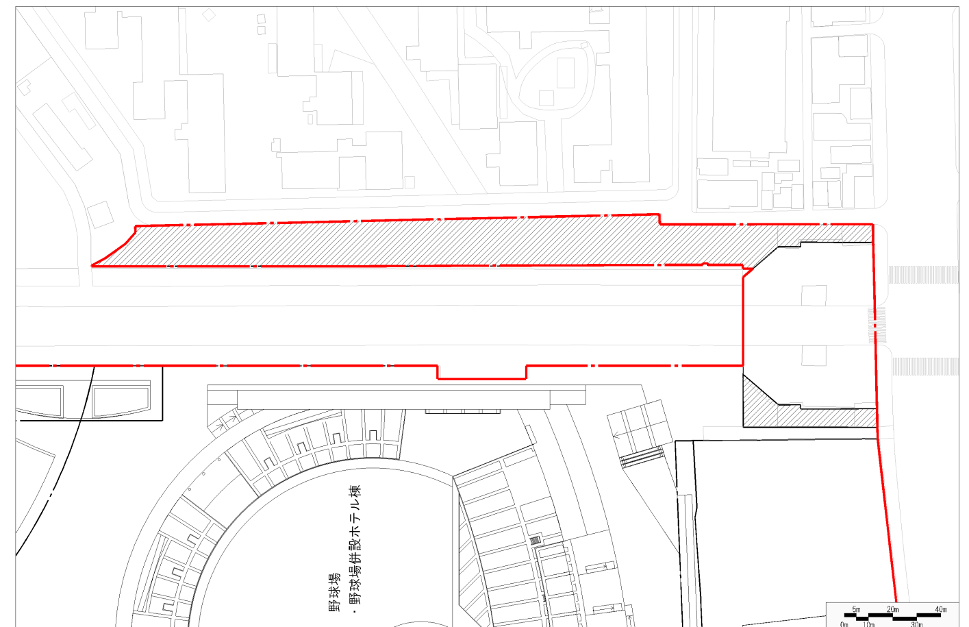
神宮外苑地区第一種市街地再開発事業 配置設計図 公共施設の設計図
